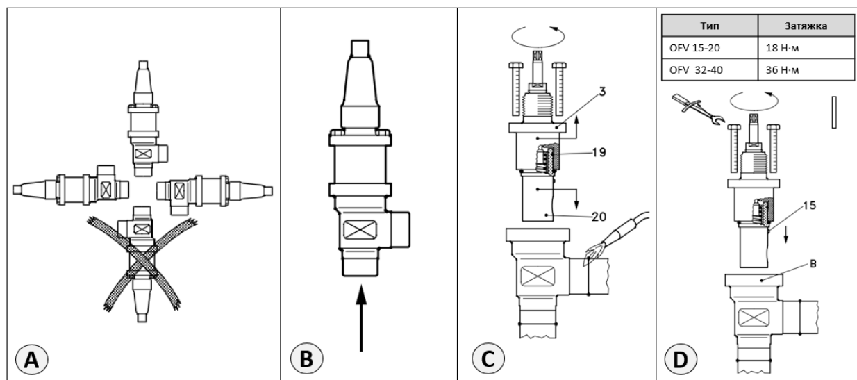
Рис. 3 – Монтаж клапана
