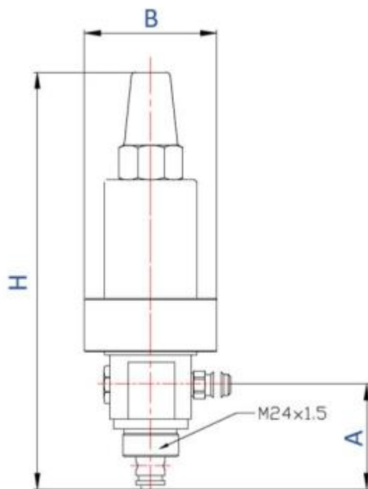
Рис. 2 – Основные размеры
