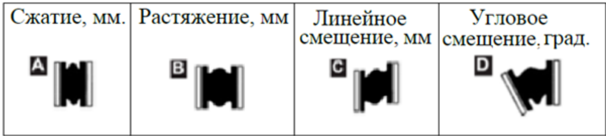
Виды деформаций гибкой вставки .
