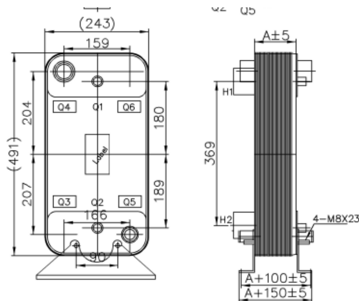
Рис.6 - Габаритные размеры и изображение теплообменника пластинчатого модификации VRHE_RD-113W
