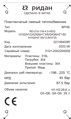
Рис.5 – Пример шильда пластинчатого паяного теплообменника BPHE
