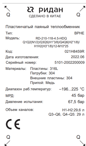
Рис.5 – Пример шильда пластинчатого паяного теплообменника VRHE
