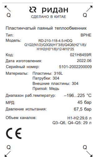
Рис.5 – Пример шильда пластинчатого паяного теплообменника БРНЕ
